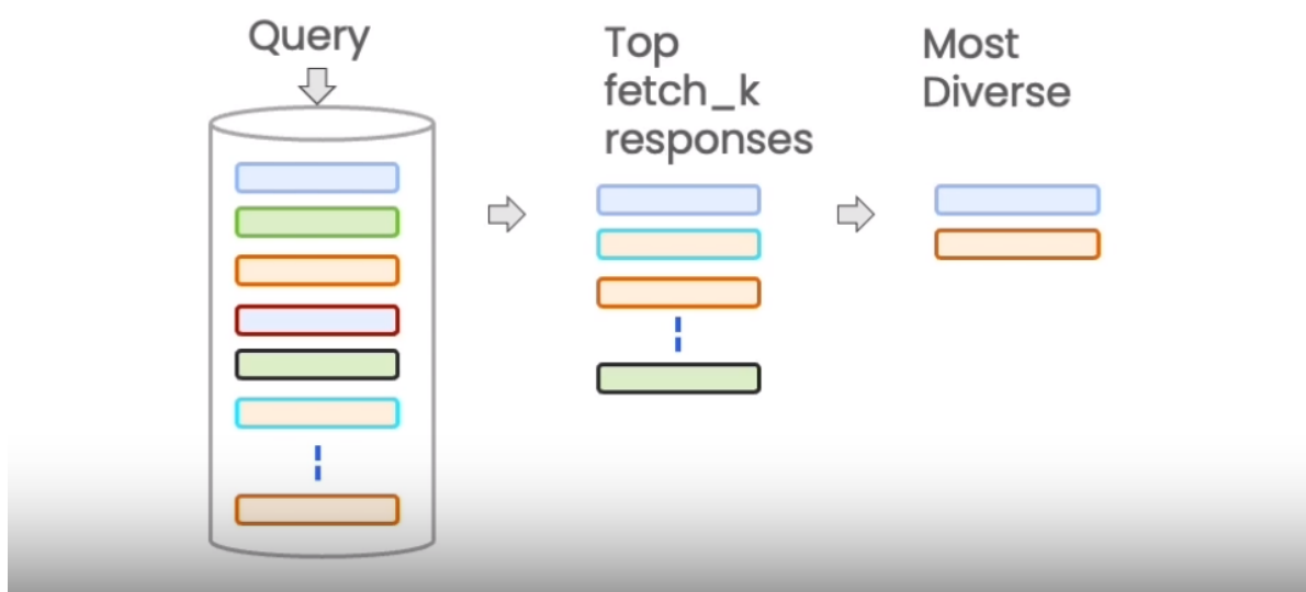
图 4.5.2 MMR
